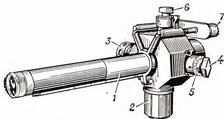
Рис. 2. Оптический прицел для прямой наводки: 1 — труба; 2 — маховик механизма углов прицеливания; 3 — барабан механизма упреждения; 4 — барашек механизма поправок направления; 5 — шкала поправок направления; 6 — барашек механизма поправок по высоте; 7 — налобник.
